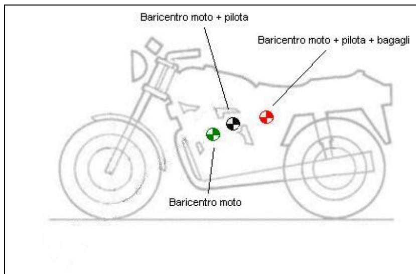
Figura 61 – Spostamento del baricentro della moto
