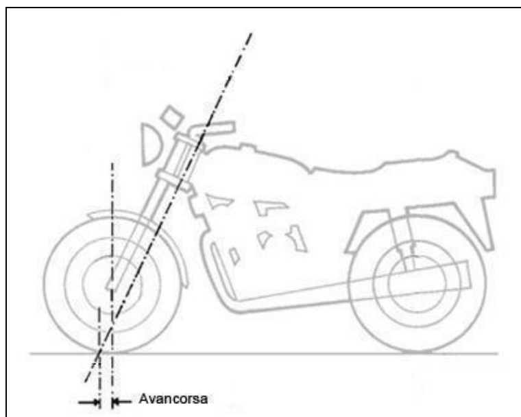
Figura 31 – Avancorsa
