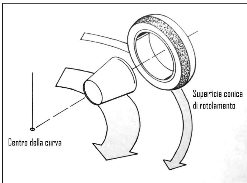
Figura 40 - Traiettoria di uno pneumatico da moto in curva
